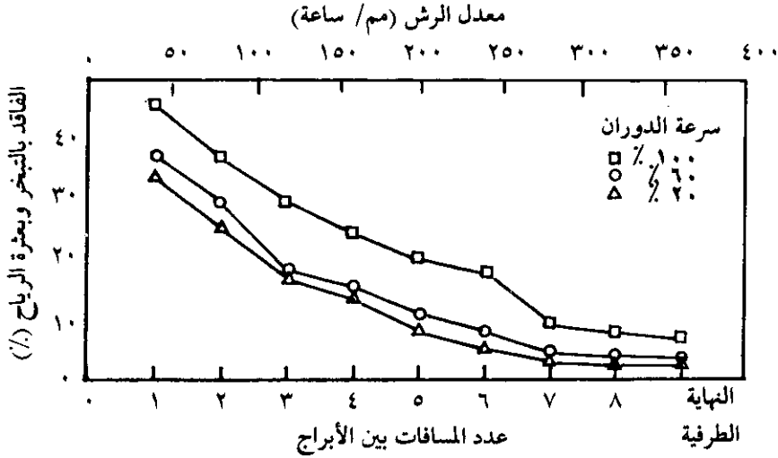
شكل رقم ٣. الفواقد بالتبخير وبعثرة الرياح لنظام الري المحوري على طول خط الرش عند سرعات دوران ومعدلات رش مختلفة.
