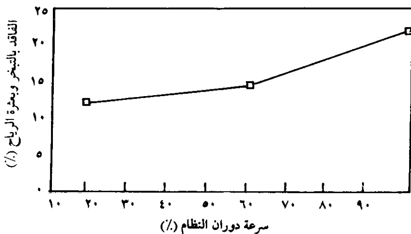
شكل رقم ٤. متوسط الفاقد بالتبخر وبعثرة الرياح تحت نظام الري المحوري عند سرعات دوران مختلفة.
