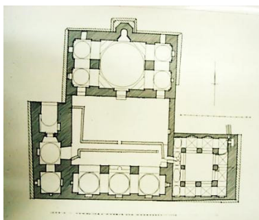
شكل (٦) مدرسة الكمالية - عن Keall
