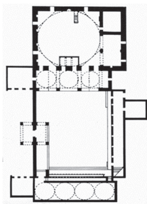
شكل (٢) جامع البكرية - عن سرجنت.
