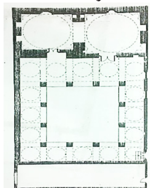
شكل (٥) مخطط مسجد جناح - عن سرجنت.
