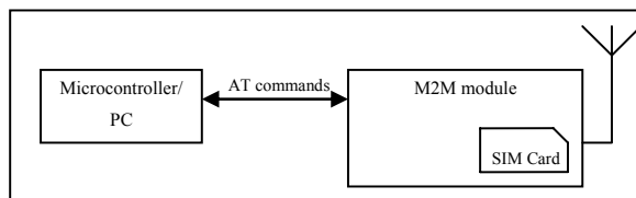
Fig. 6. M2M System.
