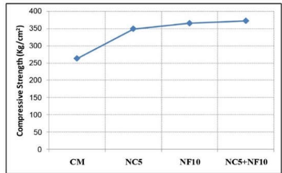
الشكل رقم (٩). اختبار الضغط لنسب استبدال نفايات الجرانيت بالرمل والأسمنت على التوالي - مرجع: (Bakhroum, 2017)
