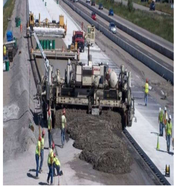
الشكل رقم (١٢). أحد الطرق التي يتم استخدامها في الرصف الأسمنتي، ويقترح البحث إضافة مادة نانو ثاني أكسيد التيتانيوم نحو بنية تحتية مستدامة المصدر: الباحث
